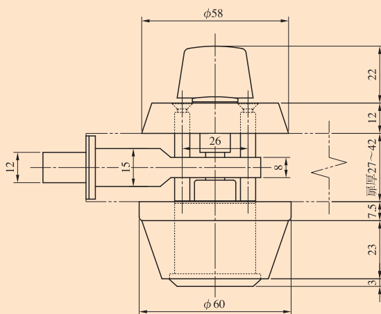
扉厚27mm以上～42mm未満の場合
