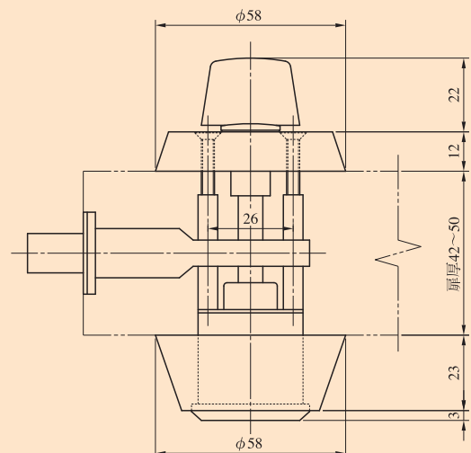
扉厚42mm以上～50mm未満の場合
