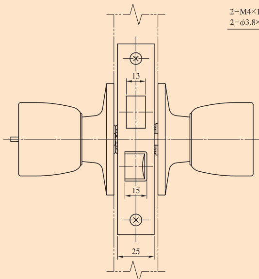
④ Nラッチバー-J型 ⑤ Nラッチバー-D型 ⑥ Nラッチバー-E型
