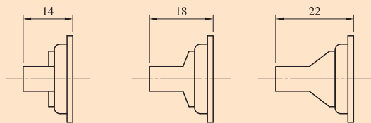
④ Nラッチバー-J型 ⑤ Nラッチバー-D型 ⑥ Nラッチバー-E型
