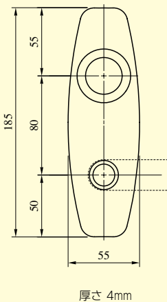
ELA15、16、17、30型を使用した場合の切欠 (ELOの場合はφ38穴が不要)
