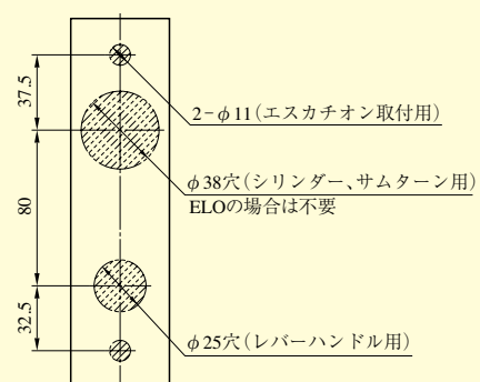
ELA15、16、17、30型を使用した場合の切欠 (ELOの場合はφ38穴が不要)
