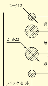
ELP13、14型を使用した場合の切欠
